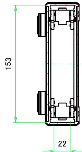
A-A (1:3)
